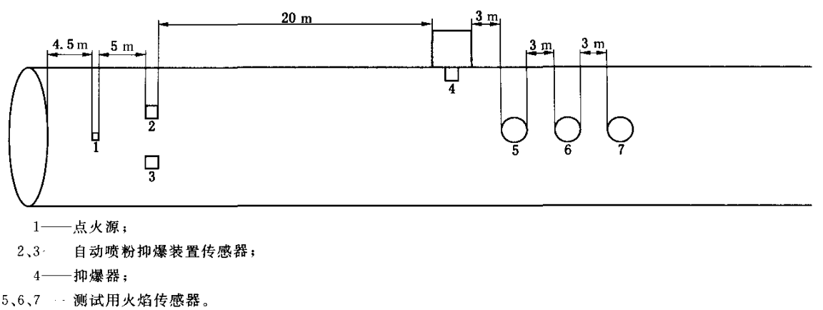
图 1 抑爆性能试验示意图
